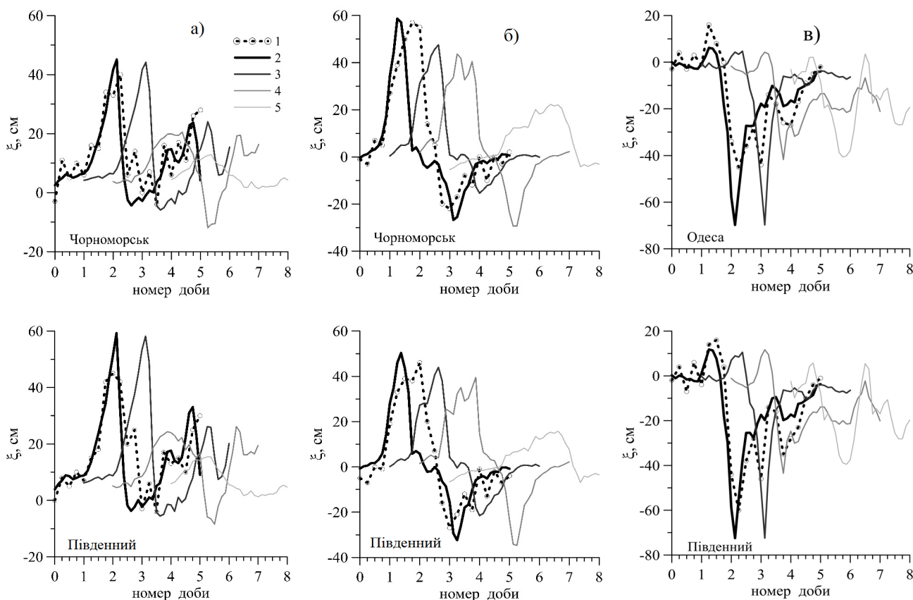
Рис. 3 – Викликані вітровою дією денівеляції рівня моря, в см, спостережені (крива 1) в портах ПнЗЧМ (а – 11.02.2016 р.; б – 13.10.2016 р.; в – 03.12.2016 р.) та отримані при прогнозуванні з різною завчасністю (криві: 2 – за 1,5-2 доби до спостереженого явища, 3 – за 3 доби, 4 – за 4 доби, 5 – за 6 діб)
