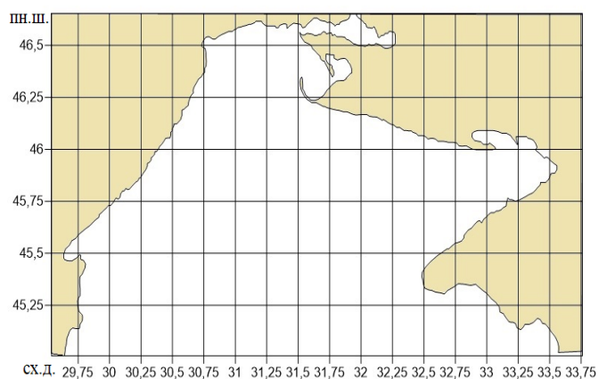
Рис. 2 – Розташування вузлів сітки GFS моделі (з просторовою дискретністю 0,25^\circ за широтою та довготою) в досліджуваній області
